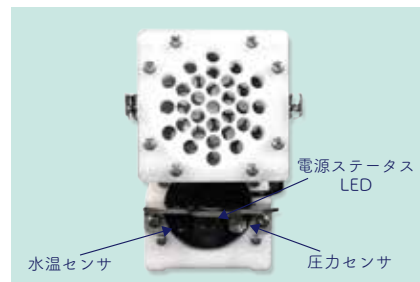
圧力センサ・水温センサ・電源ステータス LED
